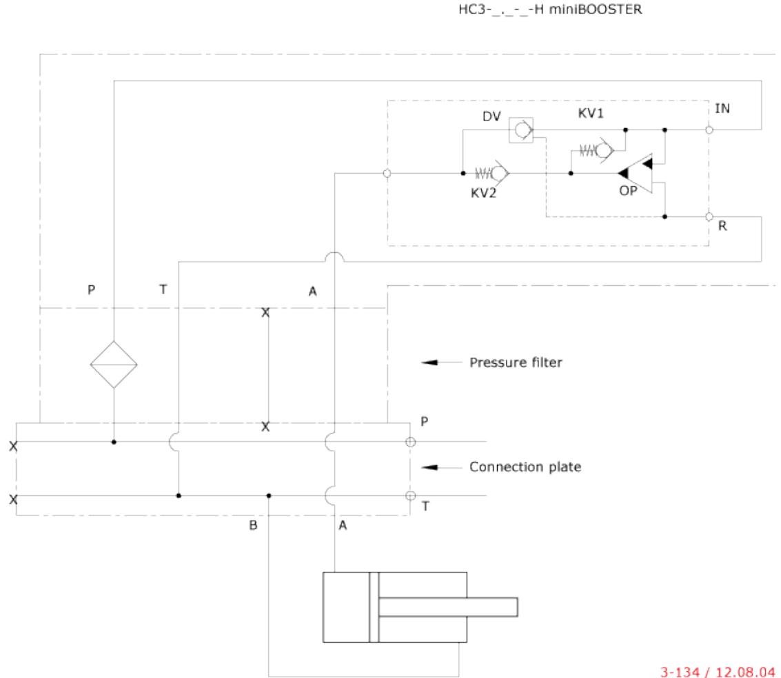
機能図
